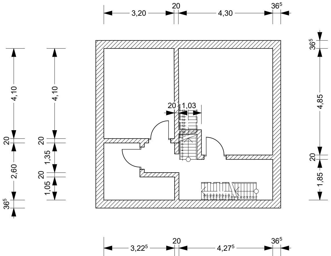
Grundrisskizze Obergeschoss
