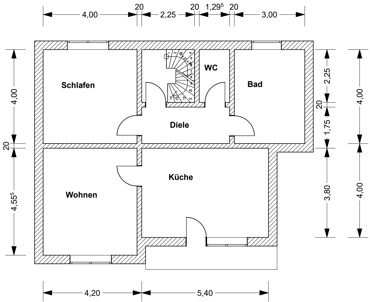
Erdgeschoss
