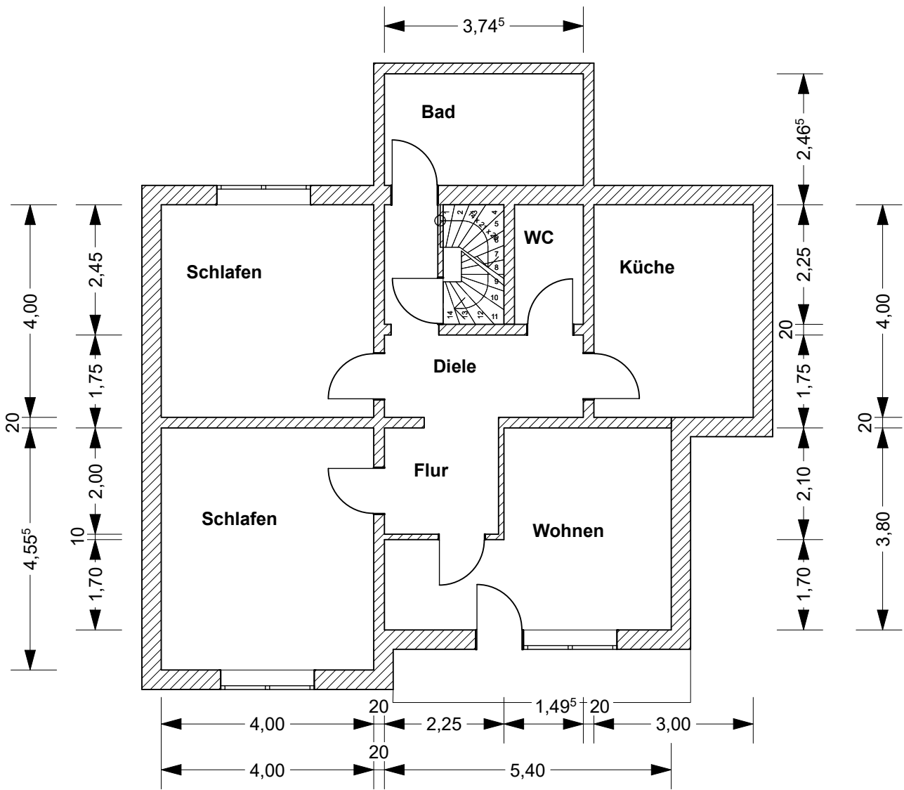
Obergeschoss
