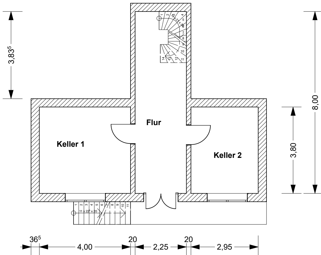
Eingangsgeschoss
