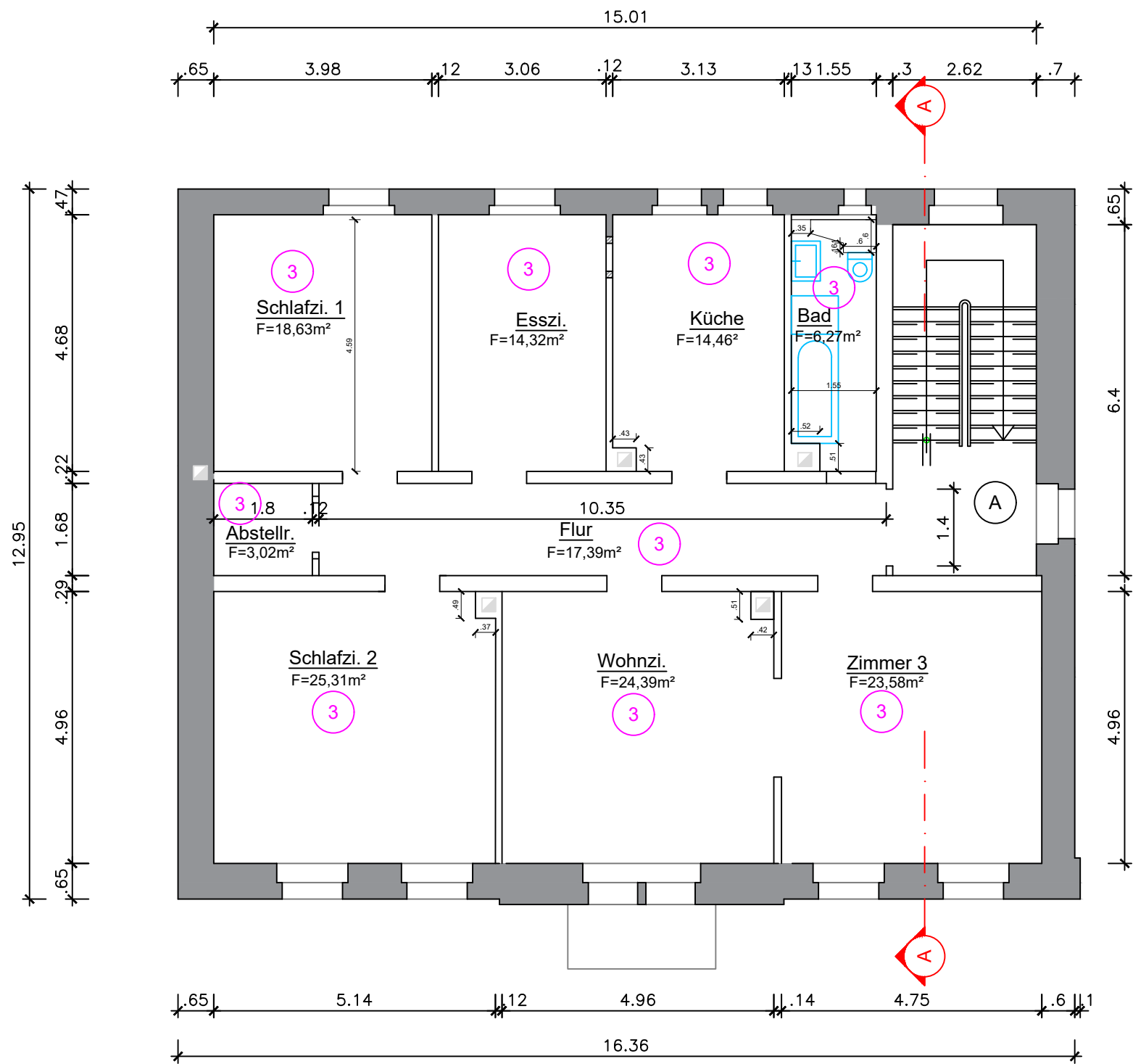
2.Obergeschoss
