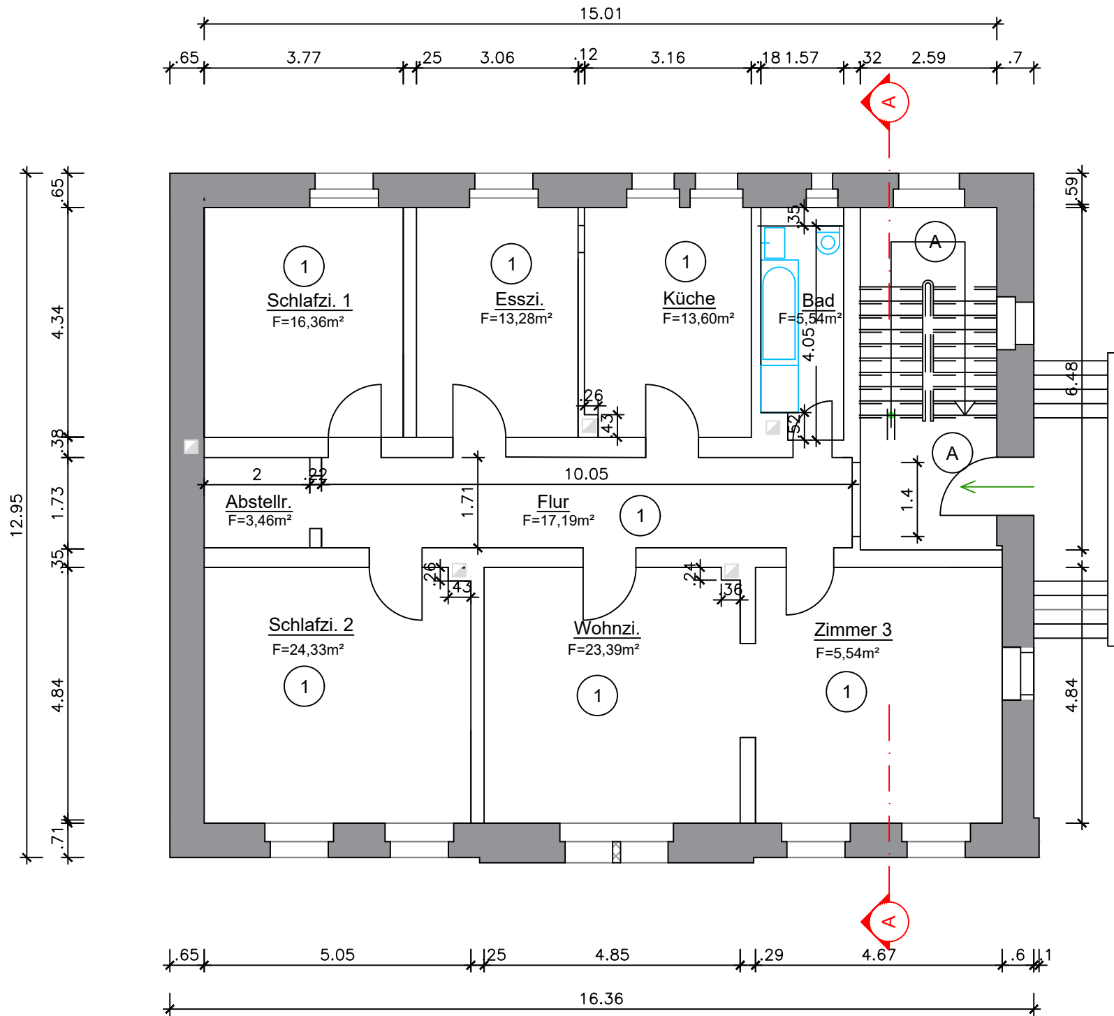
Erdgeschoss
