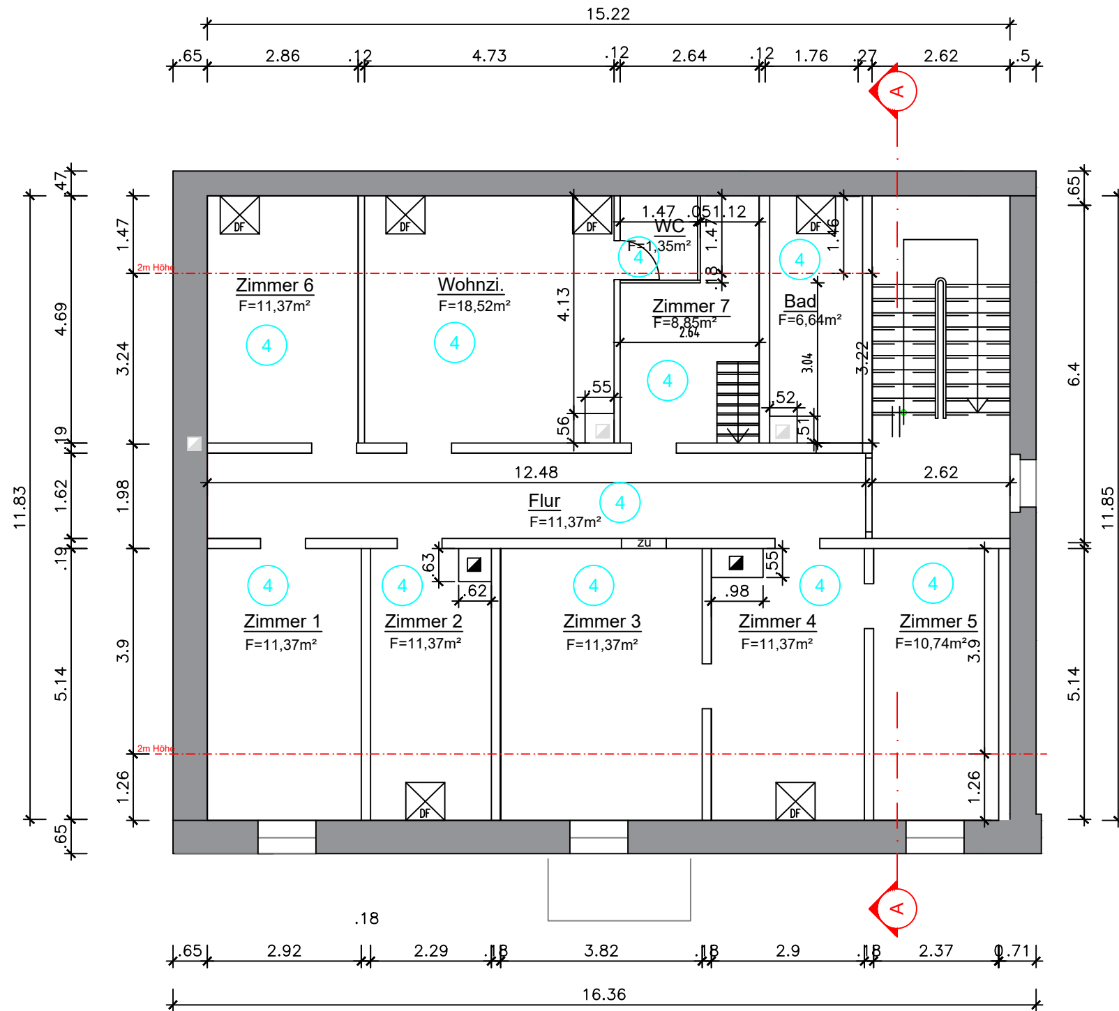
Dachgeschoss
