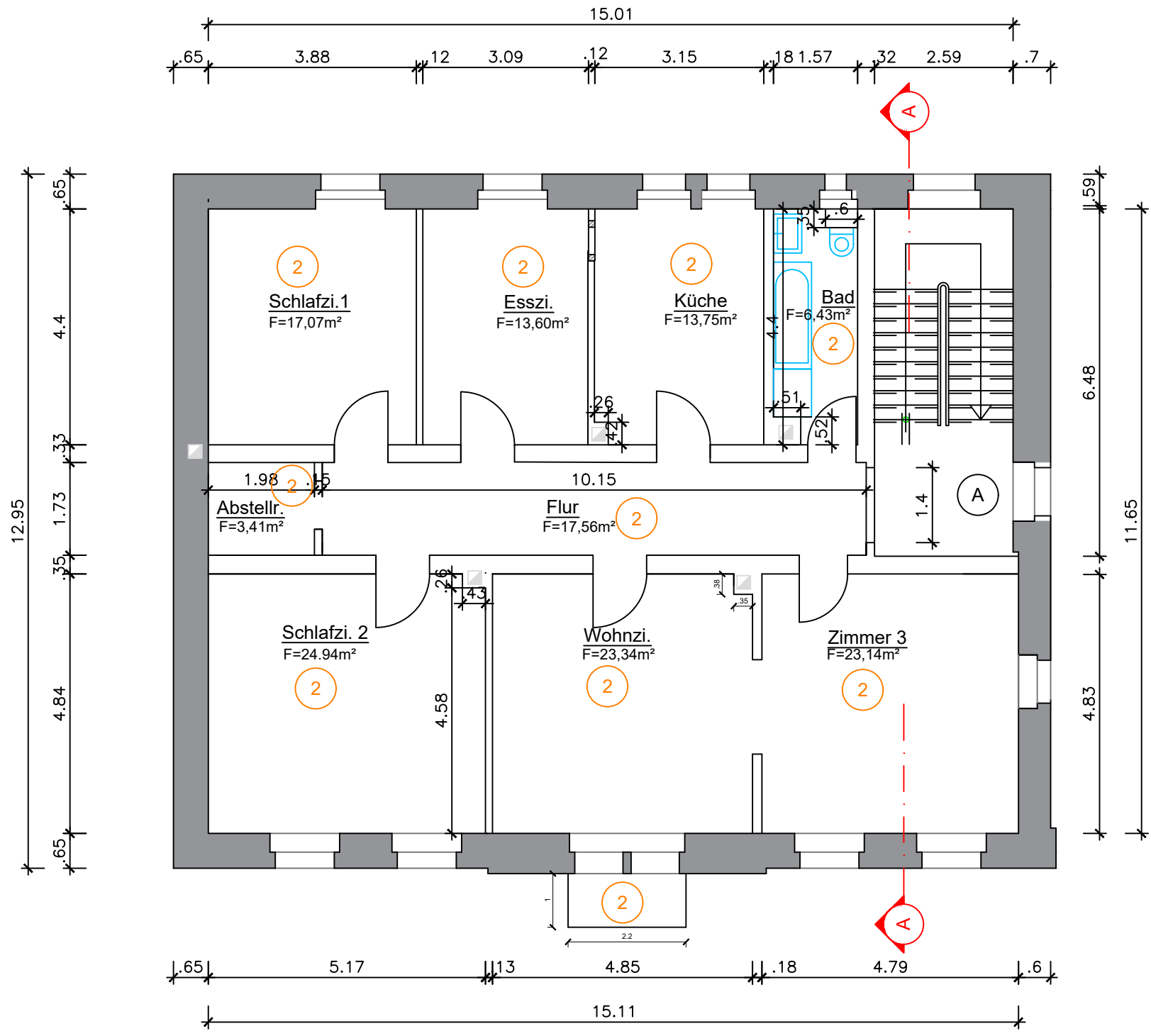
1.Obergeschoss
