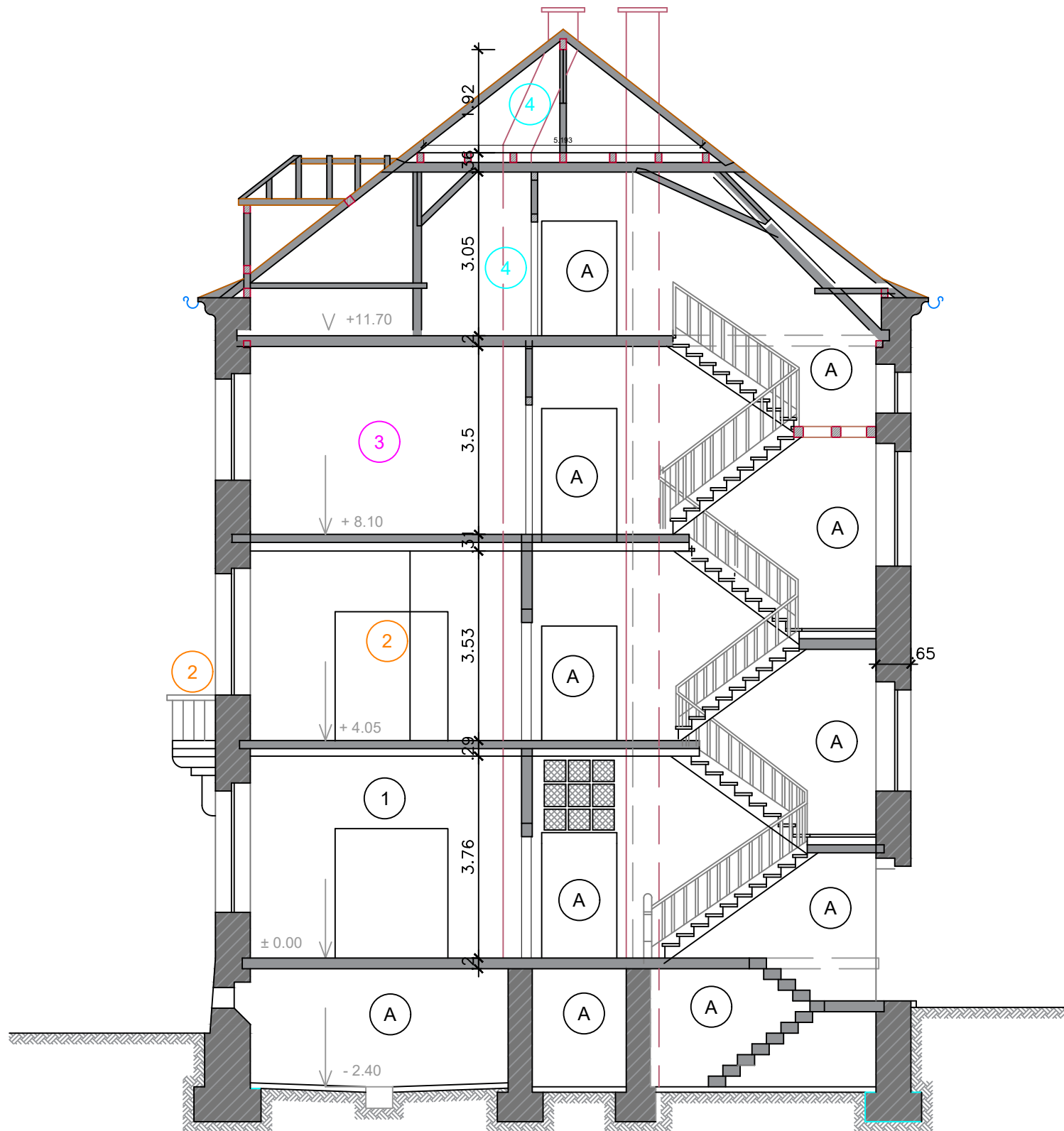
Schnitt A-A
